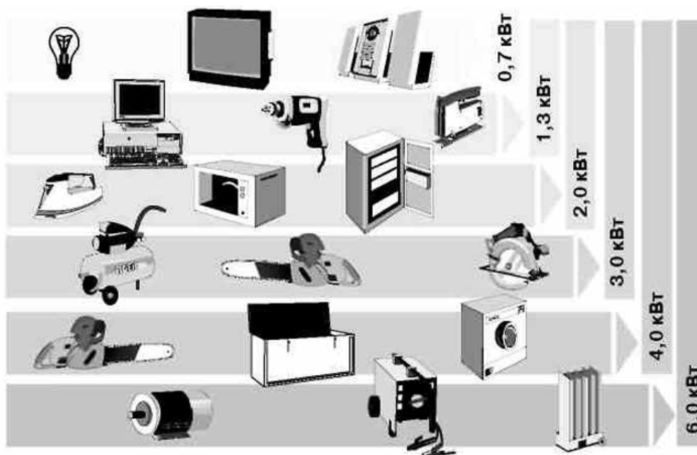
Рис. 2 Необходимая мощность электростанции при использовании наиболее распространенных бытовых электроприборов
