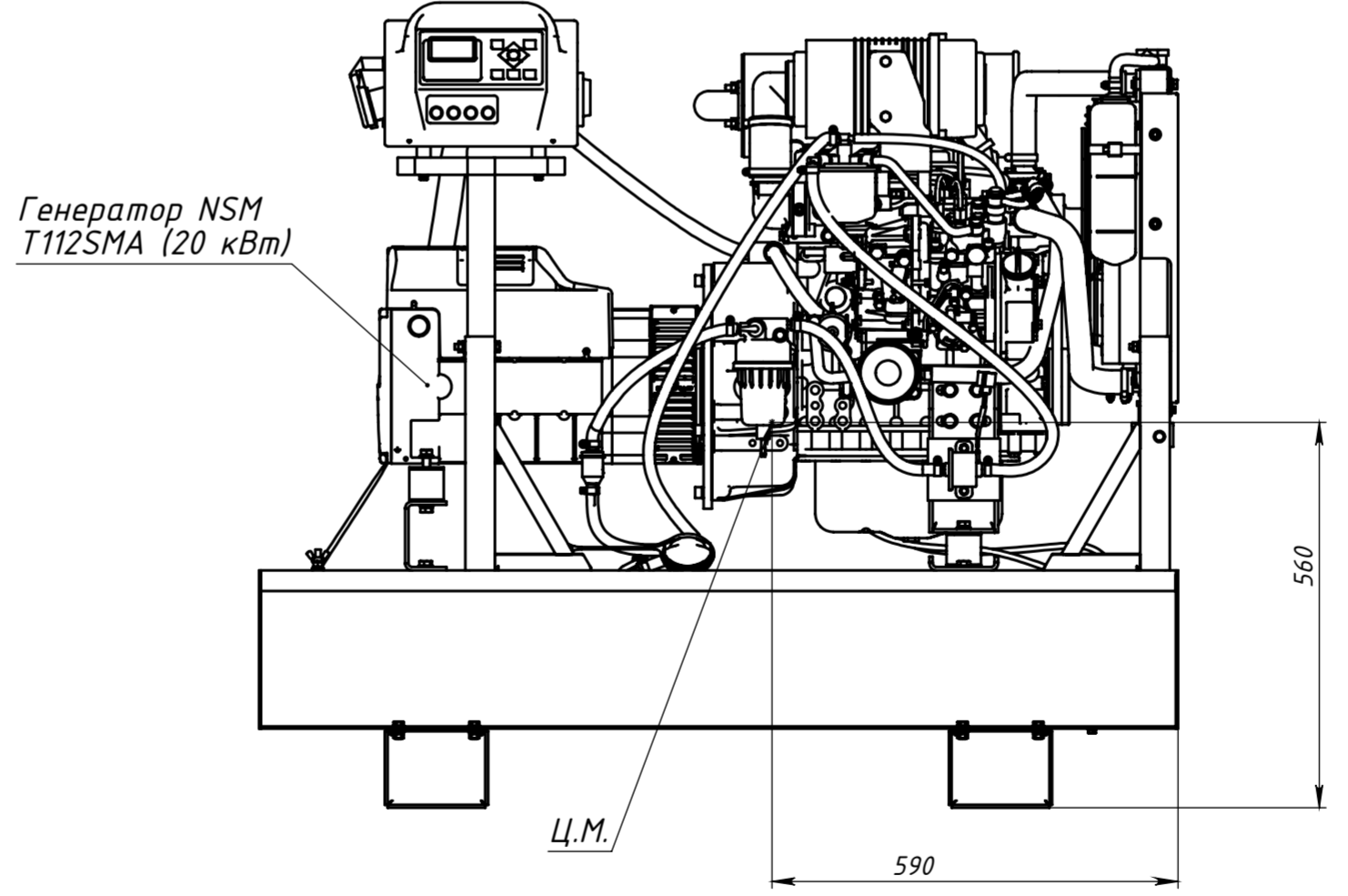
1. Размеры для справок.
