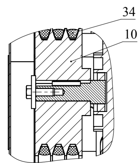
В-В (1:2.5)
