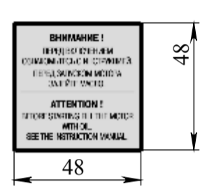
Поз.51 (1:2)
