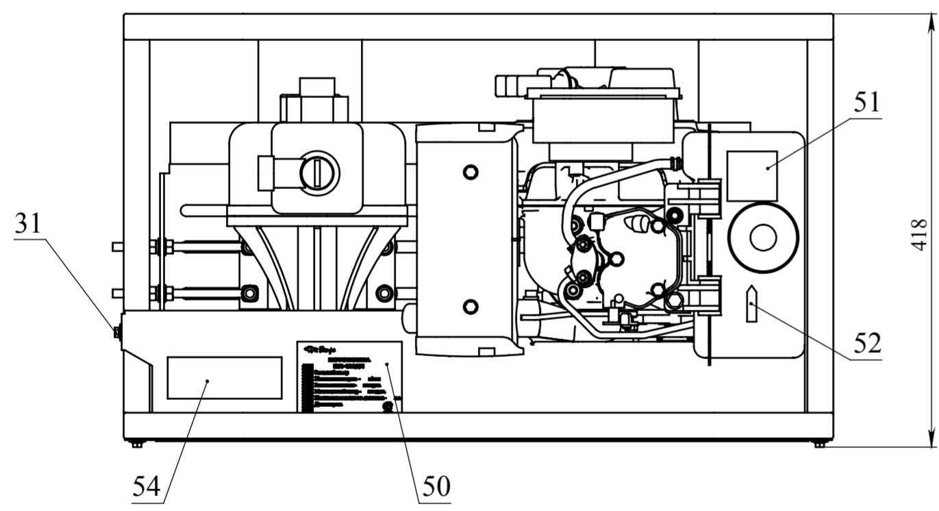
В-В (1:2.5)
