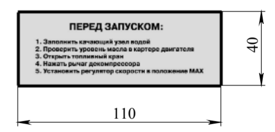
Поз.54 (1:2)
