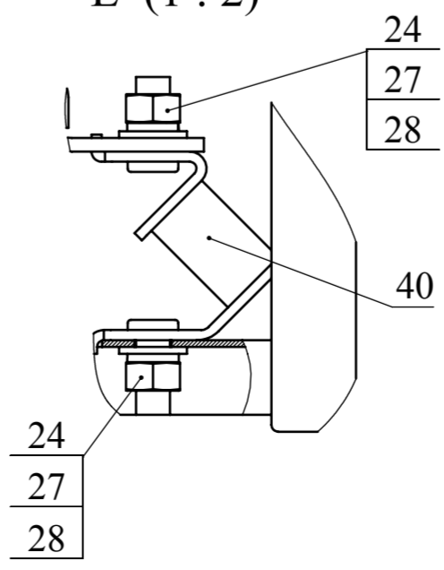
Е (1:2)
